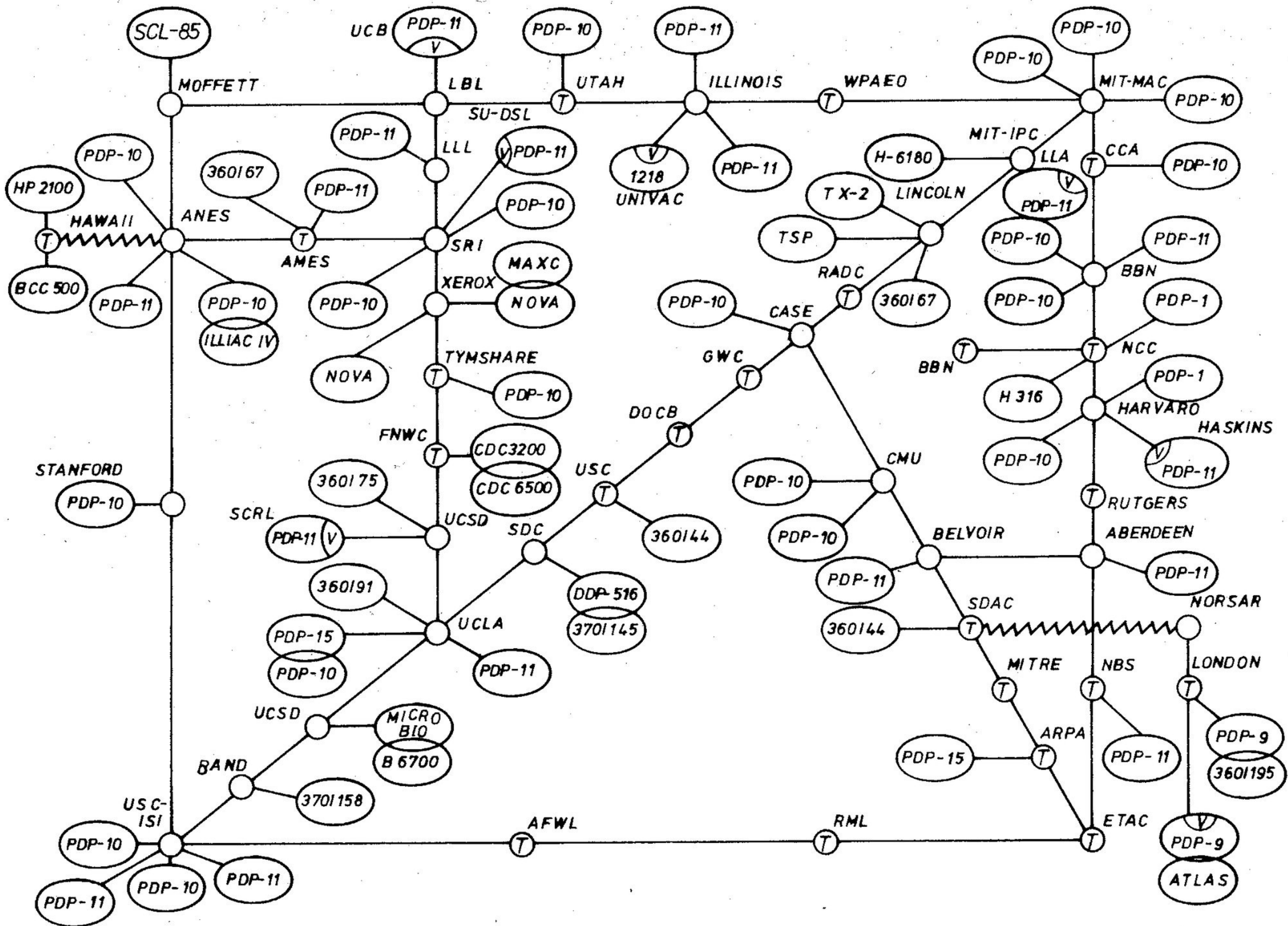
Abb. 4 ARPANET, topologische Karte. Stand Juni 1974.
